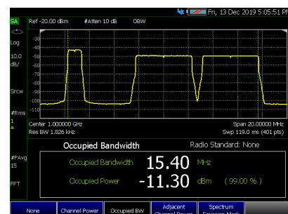
Измерение занимаемой полосы частот для сигнала LTE-A
