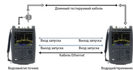
Измерение параметров кабелей большой длины с высоким уровнем потерь с помощью функции ERTA
